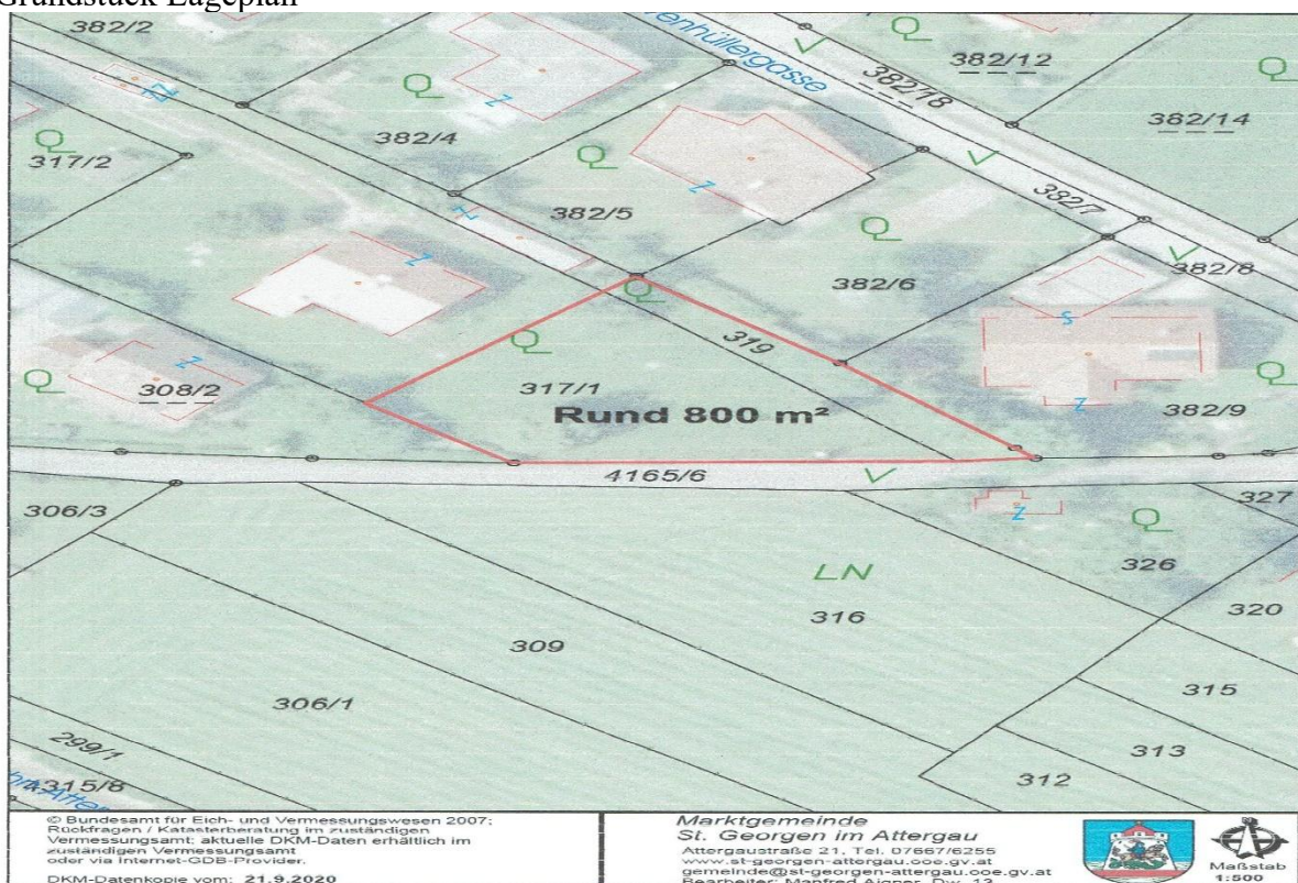
Grundstück Lageplan
